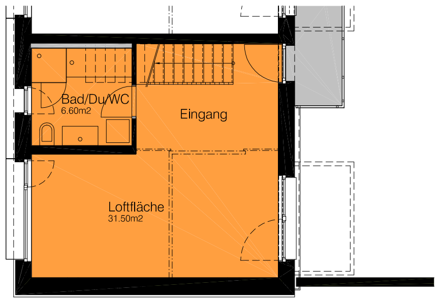
Obergeschoss
