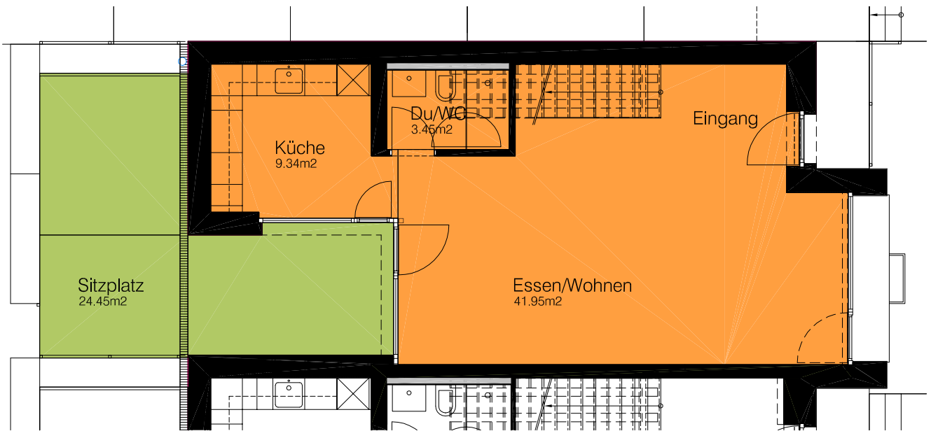
Erdgeschoss
